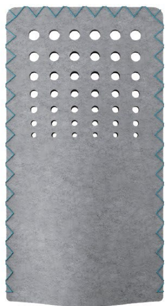
Doppler
